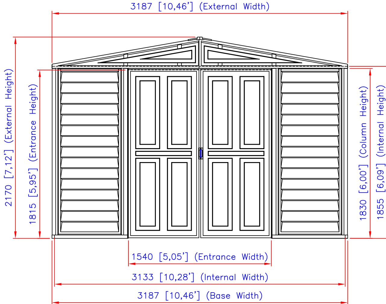
Elevation
